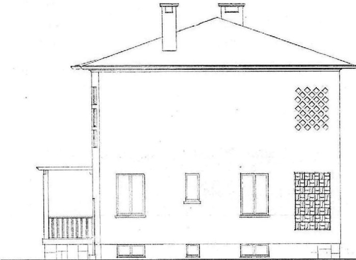
Cephe elevasyonları..
