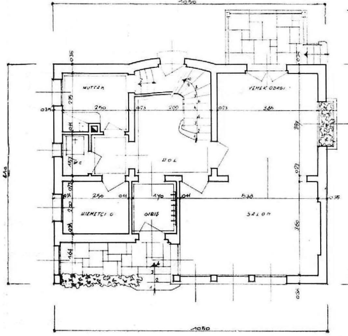
Kat plânları..
