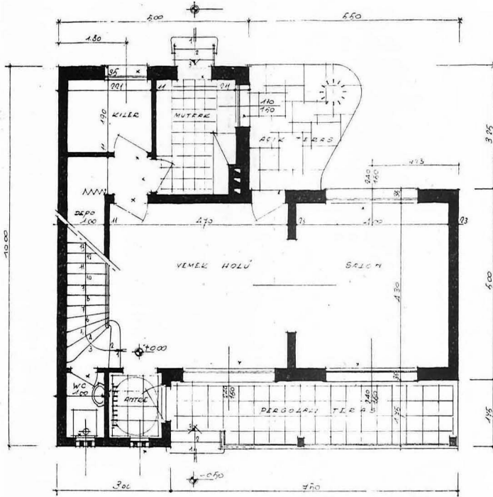
Kat plânları
